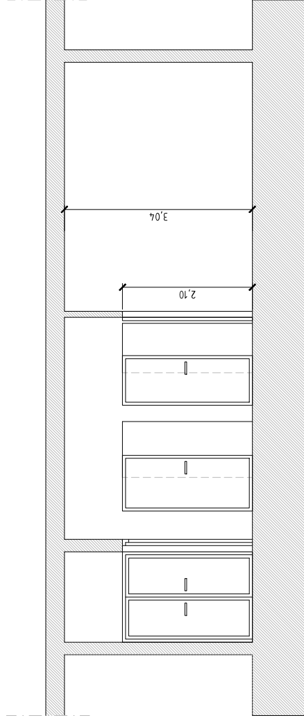
Sección 02
