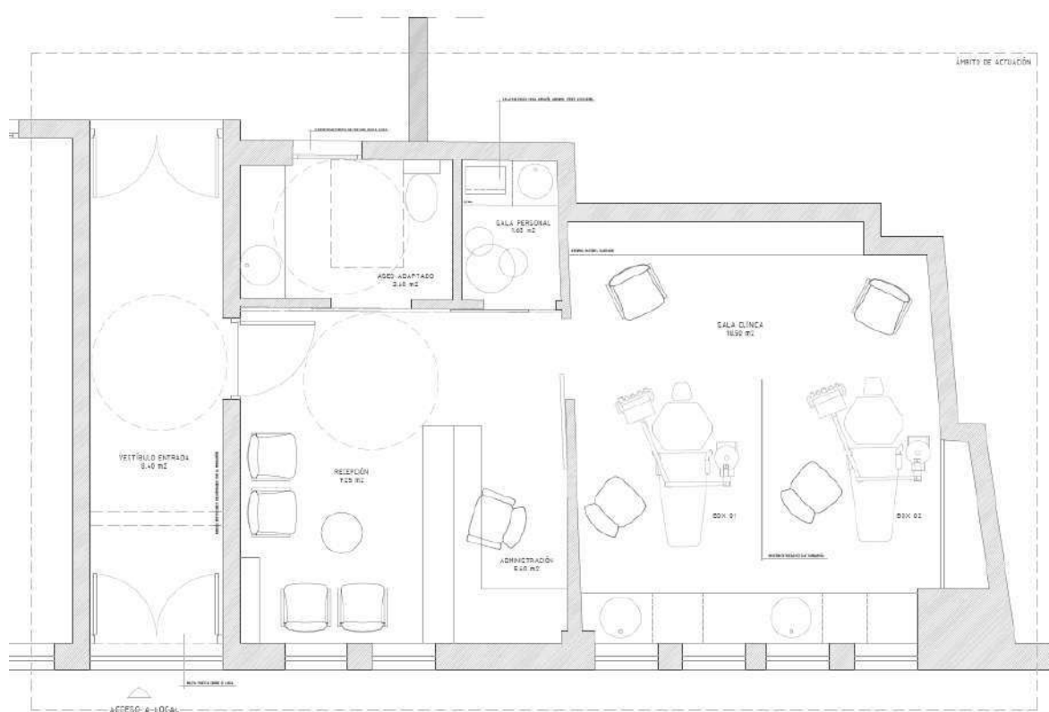
Planta reformada del local destinado a clínica dental.
